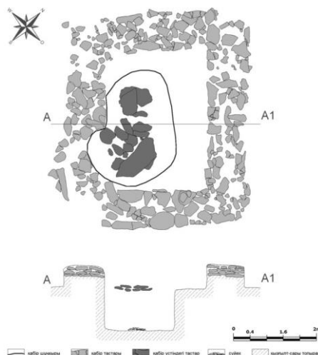
Сурет 4. Сарыоба археологиялық кешені. Қыпшақ уақытының ғибадатханасы. Қазбаның жоспары мен қимасы (Сызбаны дайындаған: А. Сералиев)
