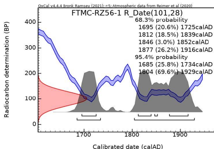
Сурет 7 – Сарыоба археологиялық кешені. №1 жерлеу орны бойынша жасалған радиокөміртегілік сараптама нәтижелері. OxCal-да есептелген калибрлеу көрсеткіштері. Радиокөміртегілік жасы 101 \pm 28 (қызыл түс), калибрлеу сызығы (көк түс) және калибрленген ықтималды уақытының мәліметтері (сұр түс).
