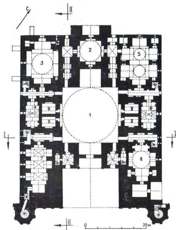
Сур. 7. Түркістан қаласындағы Қ. А. Яссауи кешенінің жобасы. Б. Т. Туякбаева бойынша [Туякбаева, 1989: 14].
